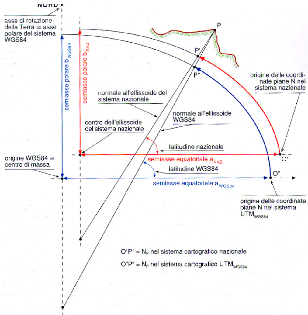
Fig.12 - Sezione meridiana sul meridiano centrale del fuso.
