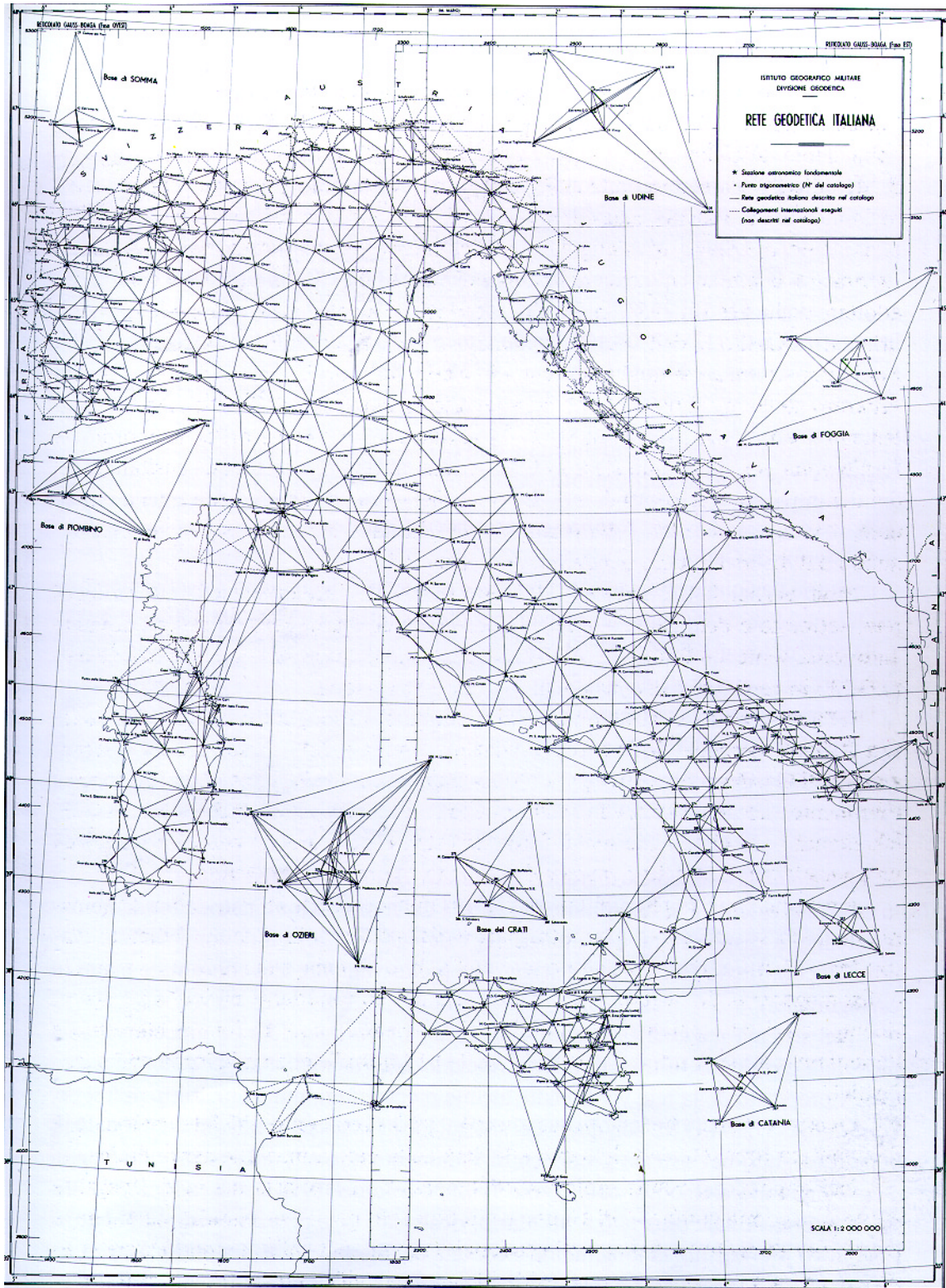
Fig. 6 – Rete geodetica fondamentale – sistema Roma40
