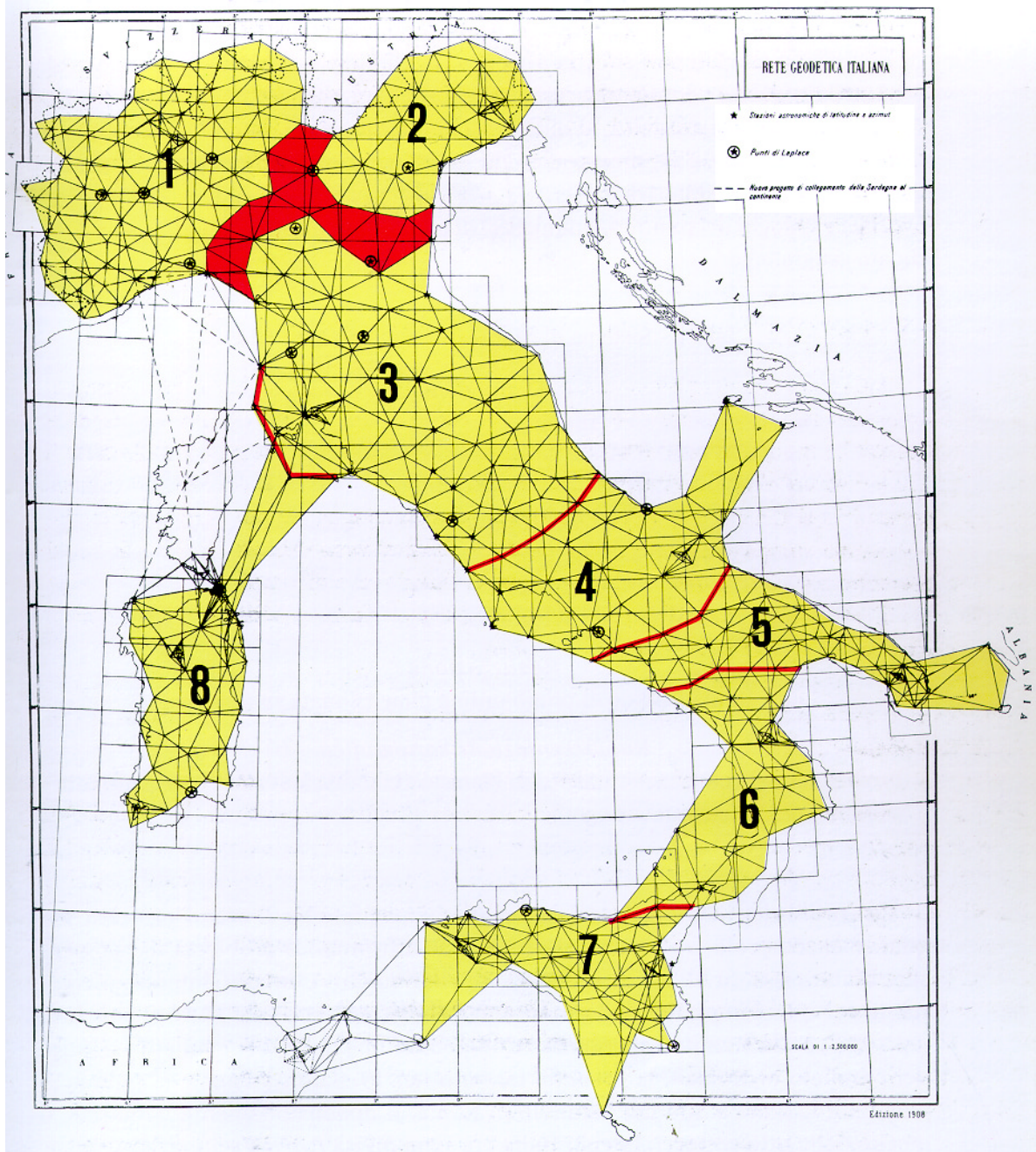
Fig. 5 - Rete geodetica fondamentale 1908-1919.
