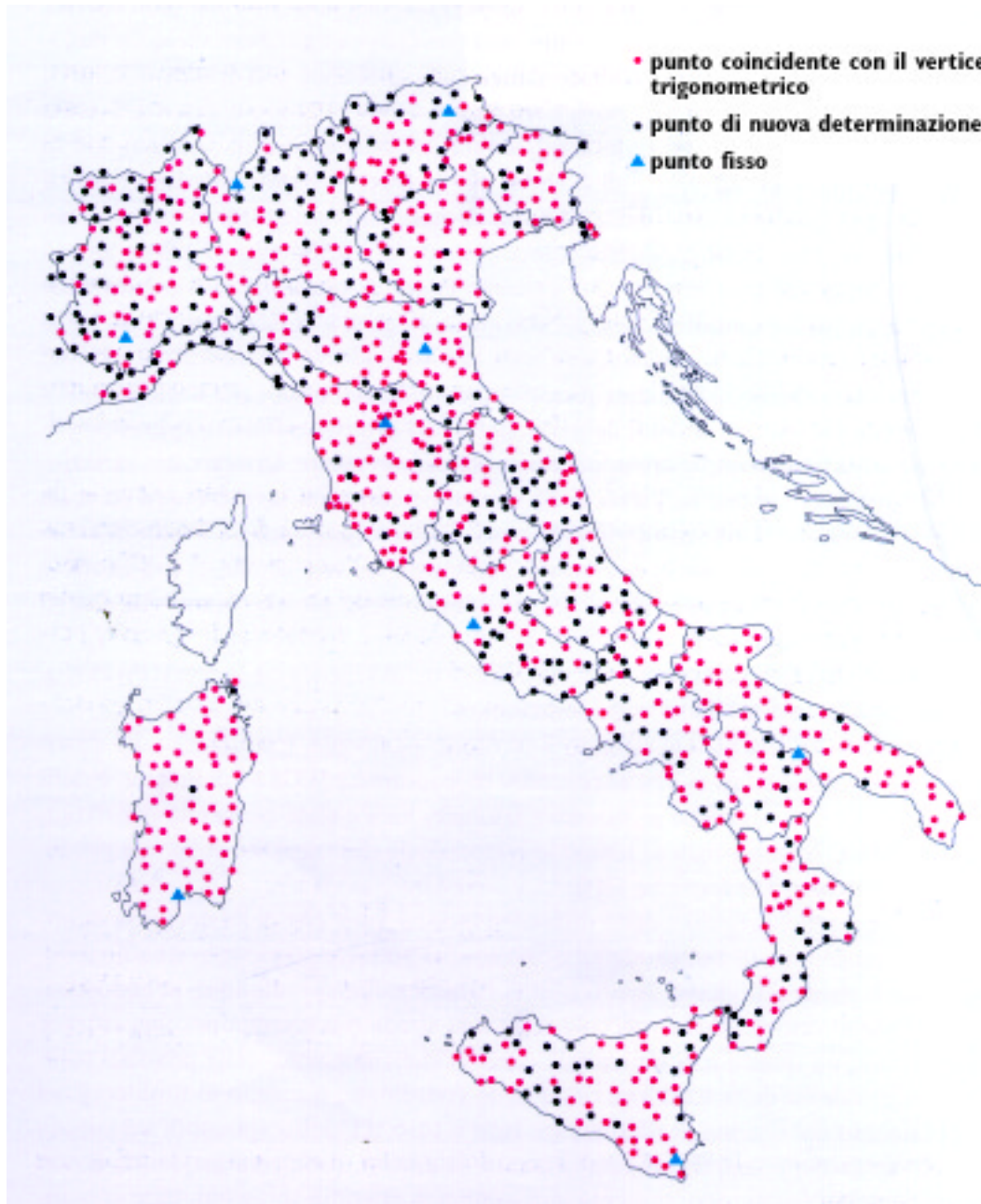
Fig.11 - La rete IGM95
